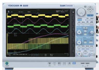
プラグインモジュール（全20種類） 本体に最大8枚のプラグインモジュールを 実装できます。
