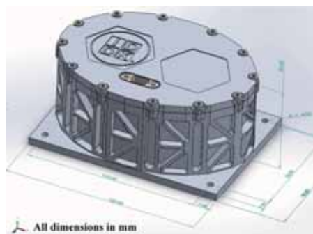
人工衛星搭載用与圧筐体
