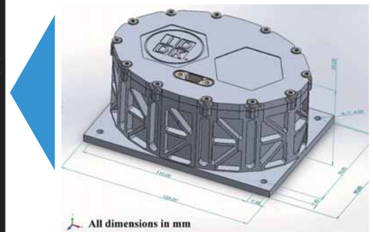
人工衛星搭載用与圧筐体
